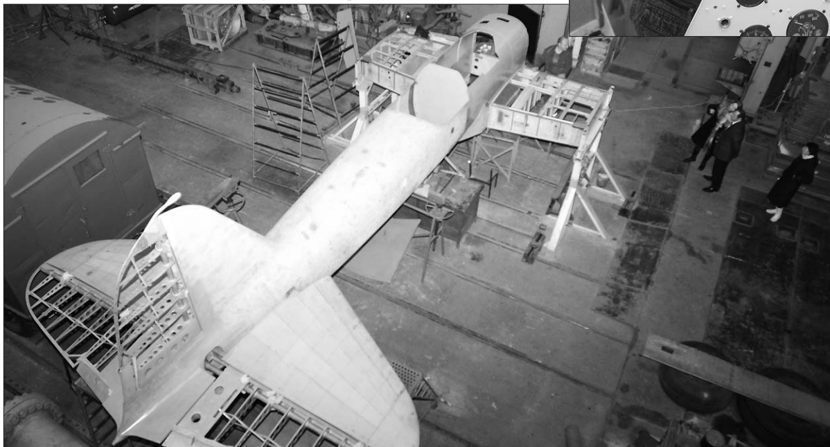
Остов Ил-2 в ангаре «Авиареставрации» «летающего танка».
